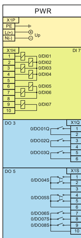
rys. 1. Karta zasilacza PWR.
