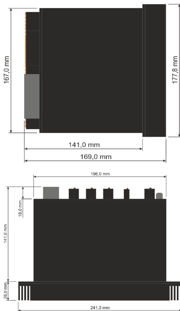
Rys. 50 Widok i wymiary urządzenia APZ-50.
