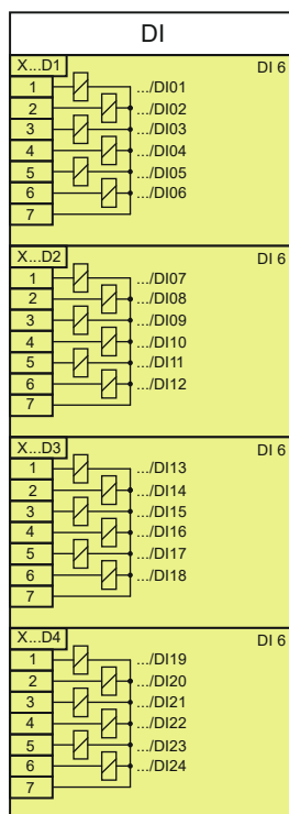
rys. 4. Karta wejść dwustanowych – DI.
