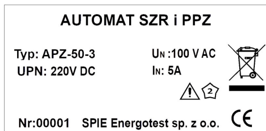
rys. 19 Tabliczka znamionowa automatu przełączania zasilania APZ-50
