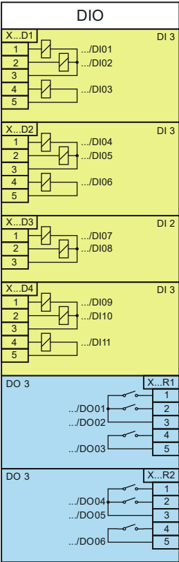
rys. 3. Karta wejść/wyjść dwustanowych – DIO.
