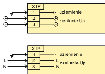
rys. 20 Schemat podłączenia zasilania automatu.
