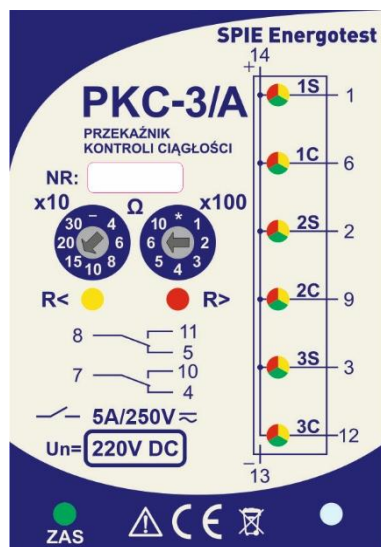
rys. 1 Front urządzenia.
