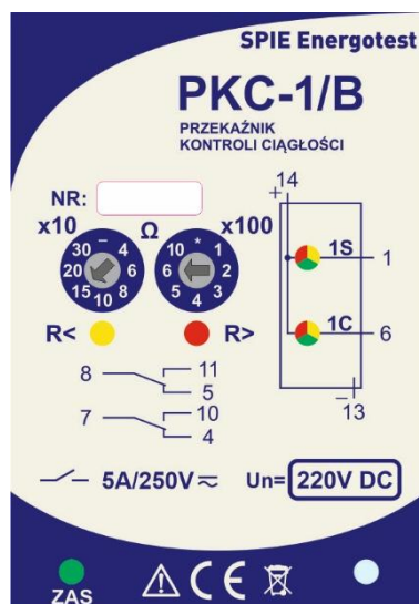
rys. 1 Front urządzenia.
